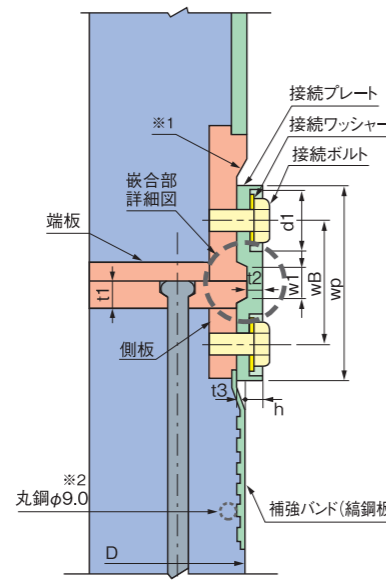
PHC杭+SC杭の例
