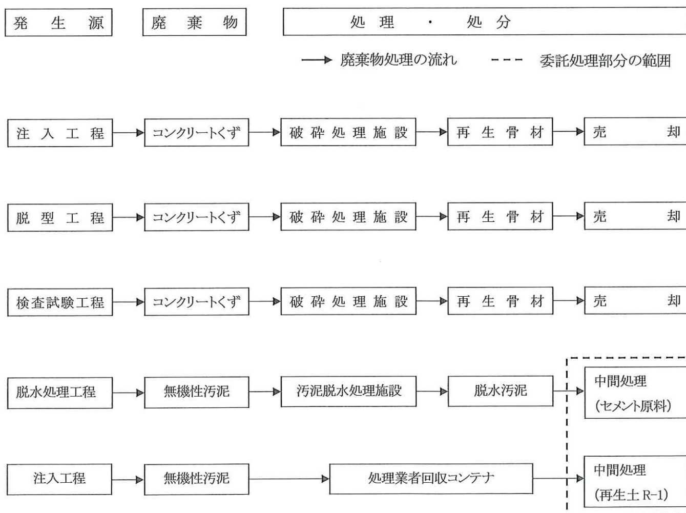
産業廃棄物処理フロー図
